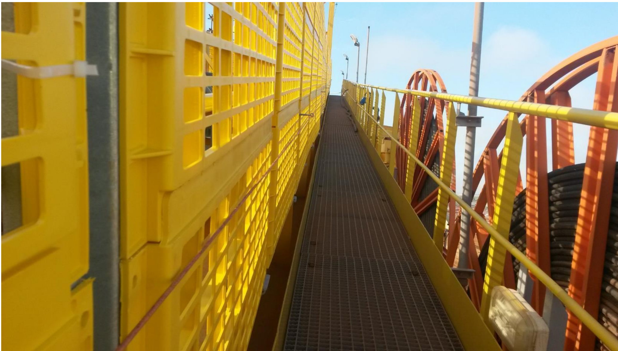
Conclusão da montagem de telas e cabo de emergência no tripper da EP-01(Lado terra)
